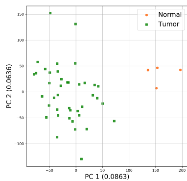
(a) PCA GSE68799
